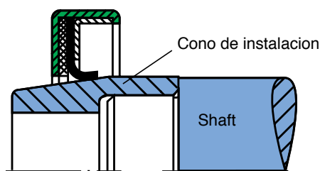
Sello de labio viendo hacia el Eje Instalación de Cono de Eje
